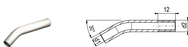
Prolunga per ugello di refrigerazione
