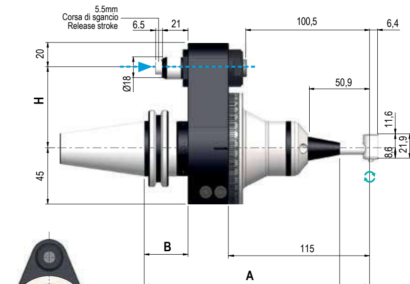
MANIPOLO ad ANGOLO 90° ANGLE SPINDLE IC - 300
