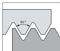
Metrisches ISO Feingewinde DIN 13 Metric ISO fine pitch DIN 13 Metrico ISO Filettatura DIN 13
